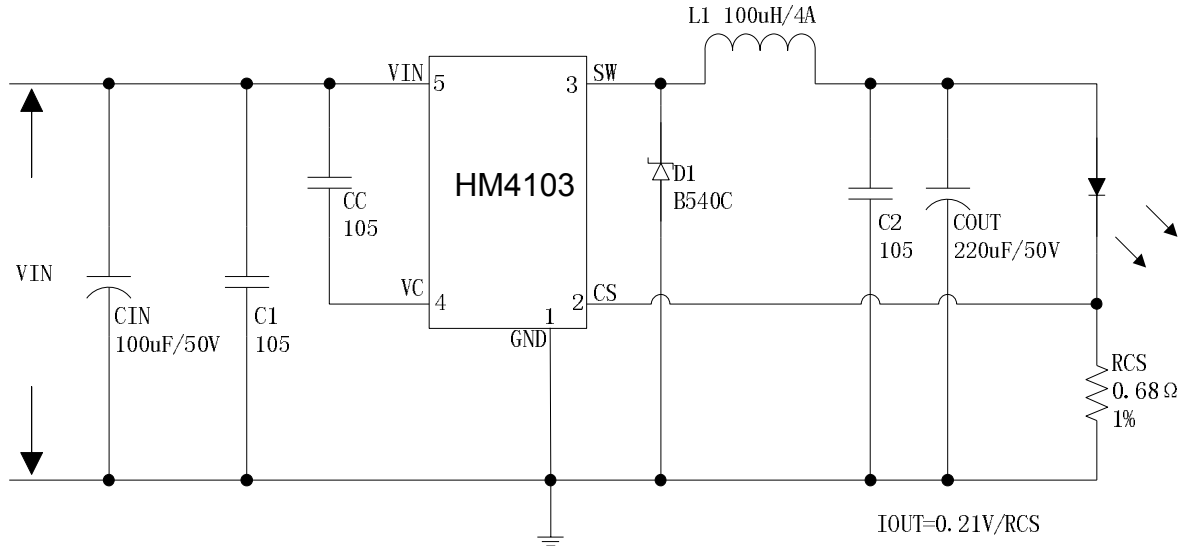
图 13.HM4103 系统参数测量电路 (VIN=8V~36V,IOUT=308mA)
