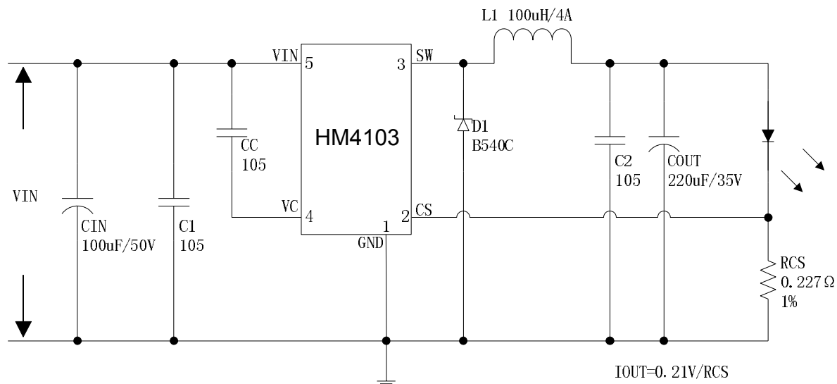
图 17. HM4103 系统参数测量电路 (VIN=8V~36V, IO UT =925mA)
