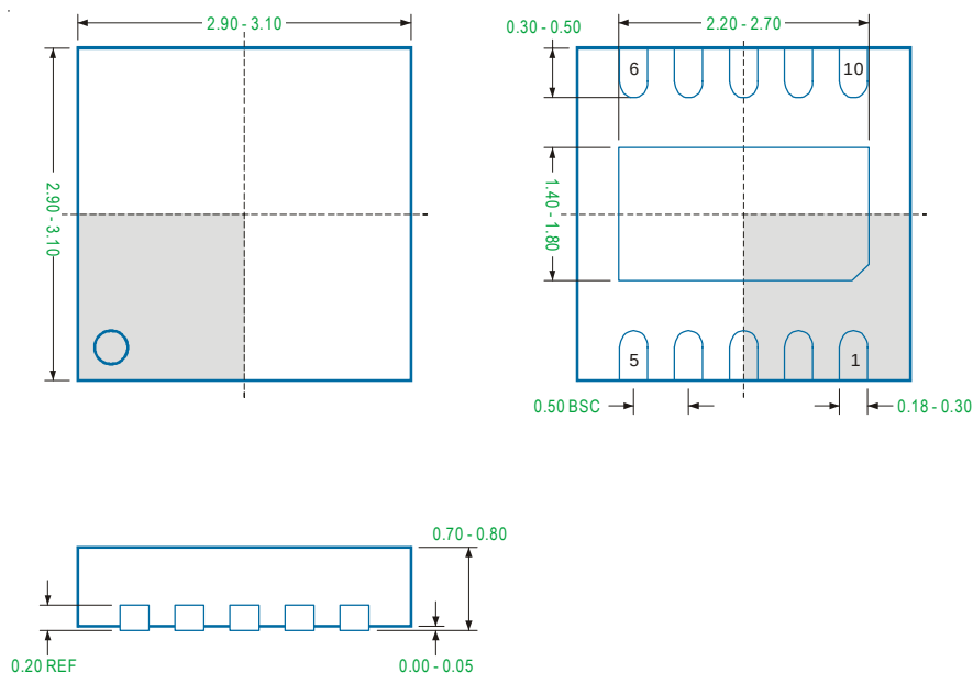
WDFN3x3-10L
