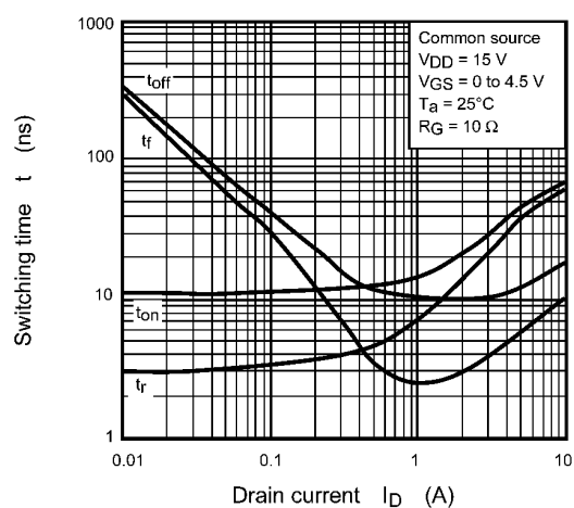
Fig. 7.11 t - I_D
