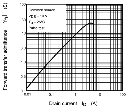
Fig. 7.8 |Y_{fs}| - I_D
