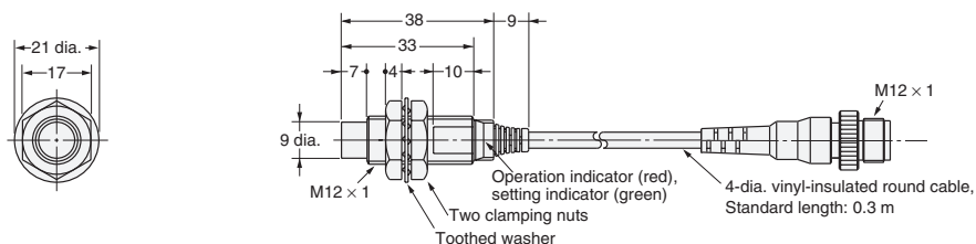
Fig. 32: E2E-X7D1-M1GJ E2E-X7D1-M1J-T
