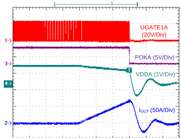
VDDA VR OCP
