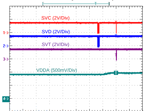
VDDA VR Dynamic VID Up
