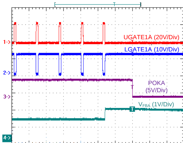
VDDA VR OVP
