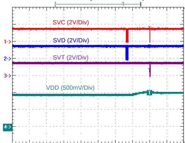
VDD VR Dynamic VID Up
