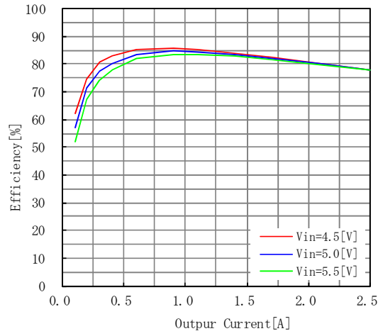
Vin=5V Vout=1.5V f=2.0MHz
