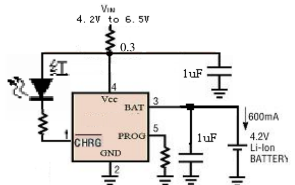
600mA 单节锂离子电池充电器
