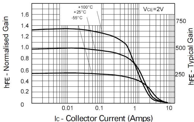
hFE v I_C
