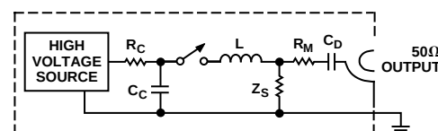
Figure 21. EFT Generator
