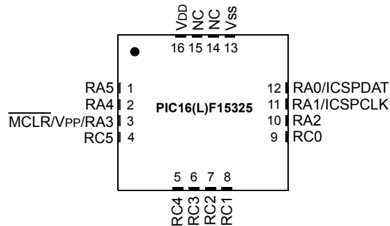
16-PIN UQFN/VQFN/QFN (4X4)
