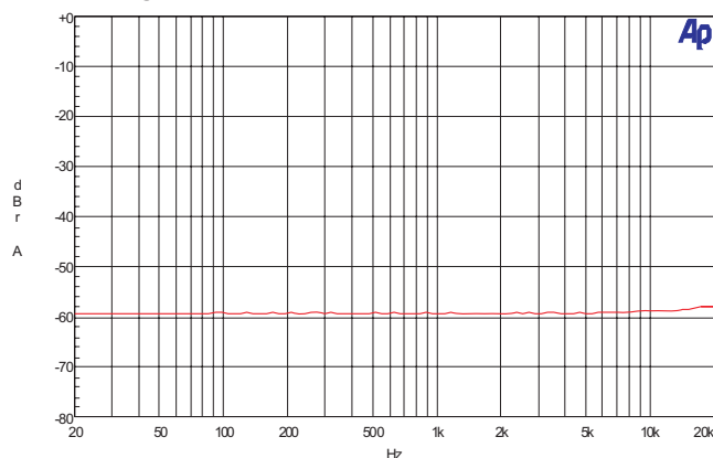
11. CMRR
