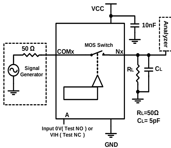
Figure4. Off Isolation ( V_{ISO} )
