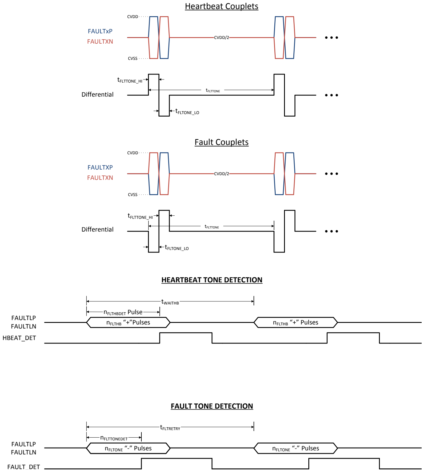
图 31. FAULT Tones
