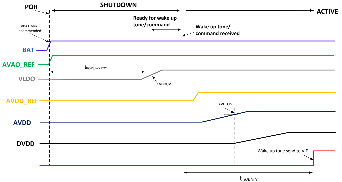
图 2. Startup Diagram
