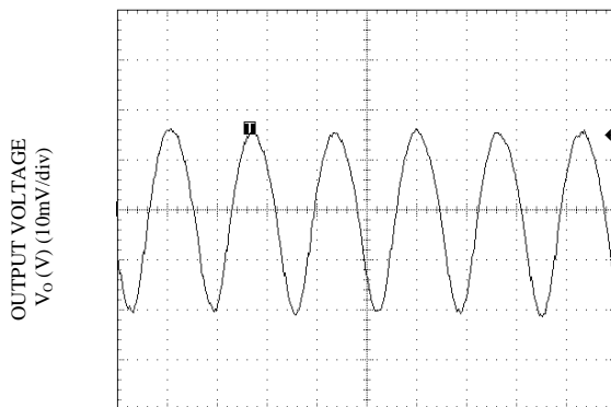
Vin=12V, Vo=1.8V, Io = Io,max
