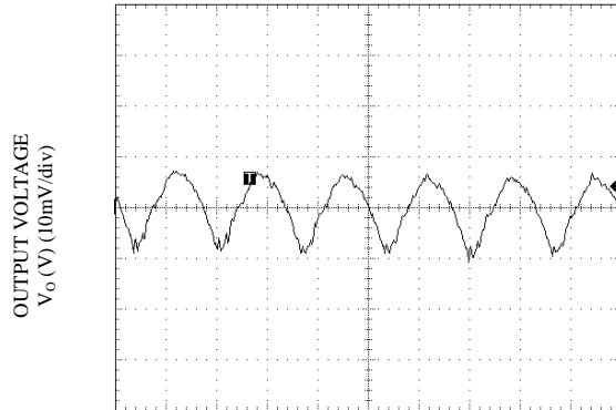
Vin=12V, Vo=1.2V, Io = Io,max
