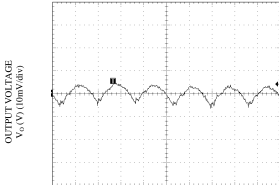
Vin=12V, Vo=0.6V, Io = Io,max
