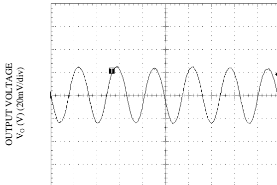
Vin=12V, Vo=2.5V, Io = Io,max
