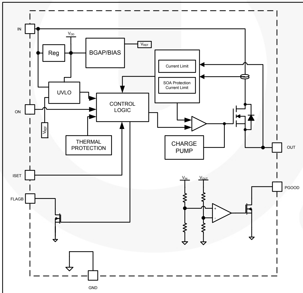
图 5. 框图
