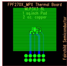
图 8. 80 ^\circ\text{C/W} , 安装在一个 2-oz 的 1in 2 焊盘上铜
