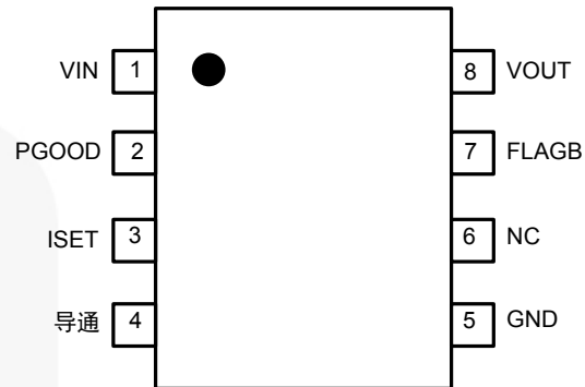
图 7. SO8（俯视图）
