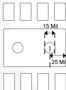
图 41. 内嵌在 DAP 中的两个通孔式过孔
