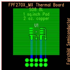
图 10. 102 ^\circ\text{C/W} , 安装在一个 2-oz 的 1in 2 焊盘上铜
