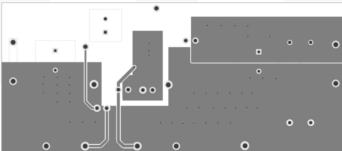
图 45. 底视图和 ASB 层
