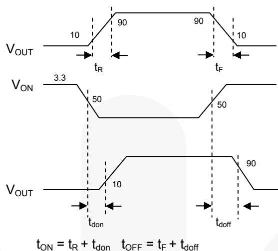
图 12. 时序图
