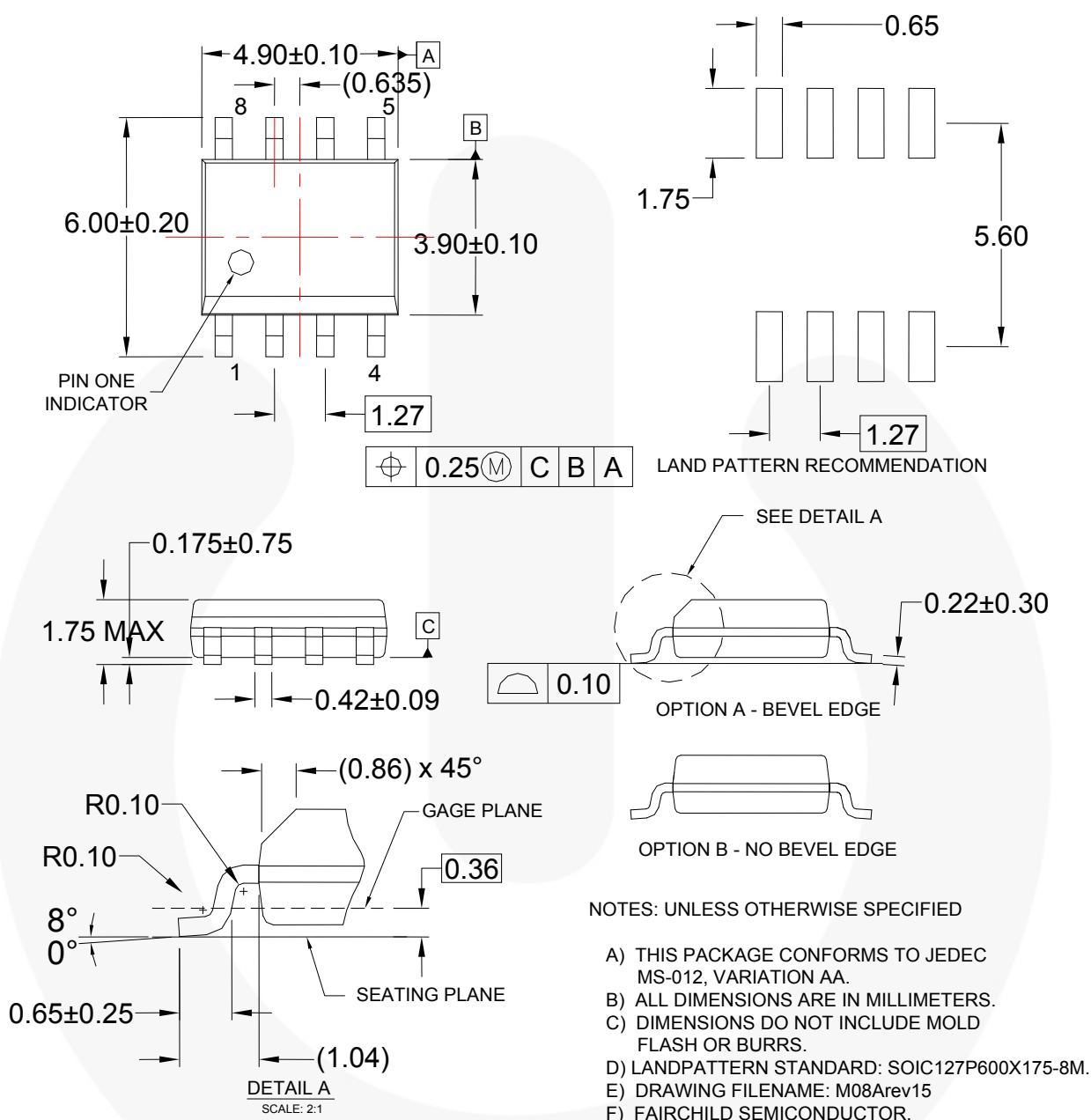
图 46. 8-引脚式小尺寸封装 (SOP)
