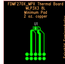
图 9. 226 ^\circ\text{C/W} , 安装在一个 2-oz 的最小焊盘上铜
