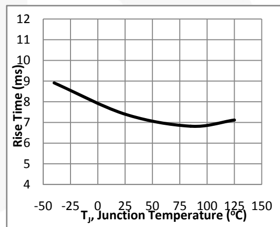
图 20. 输出上升时间和结温
