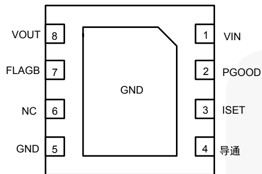
图 6. MLP（底视图）
