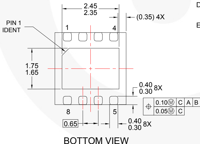
图 47. 8 引脚, 3x3 mm 模塑无铅封装 (MLP)
