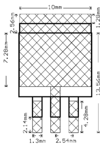
TO-263T
