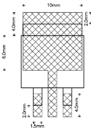
TO-263
