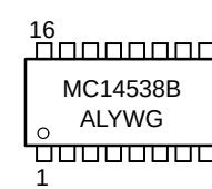
SOEIAJ-16
