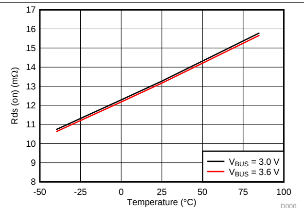
图 6. R_{ds(on)} vs Temperature
