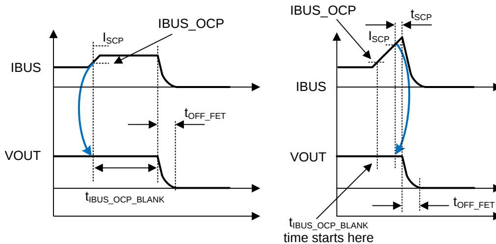
图 11. IBUS OCP and SCP
