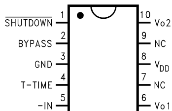
Mini Small Outline (MSOP) Package
