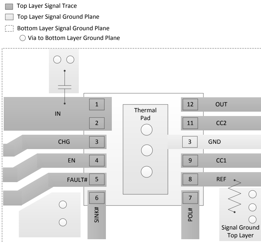
图 22. Layout Example
