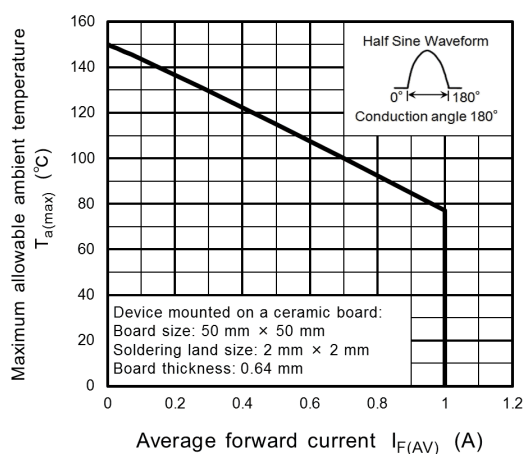
Fig. 10.3 T_{a(max)} - I_{F(AV)}
