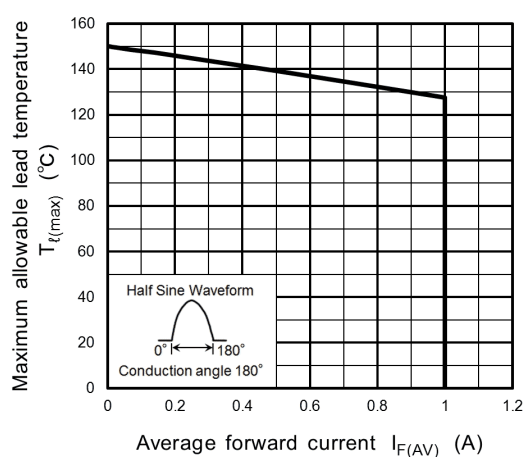
Fig. 10.5 T_{l(max)} - I_{F(AV)}
