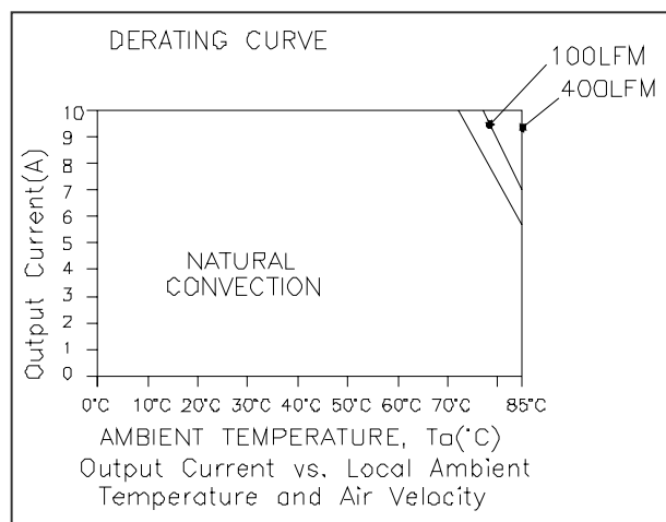
S7BC-10E2Ax, V_o=1.8\text{V}
