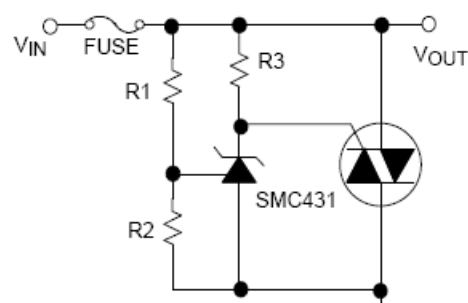
Fig. 23 Crow Bar
