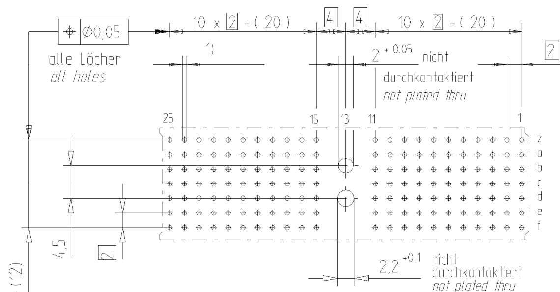
Lochbild für Leiterplatte (Bestückungsseite)
