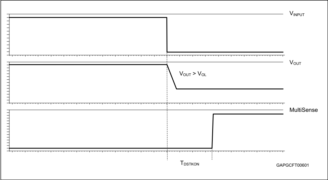
Figure 4. T_{DSTKON}
