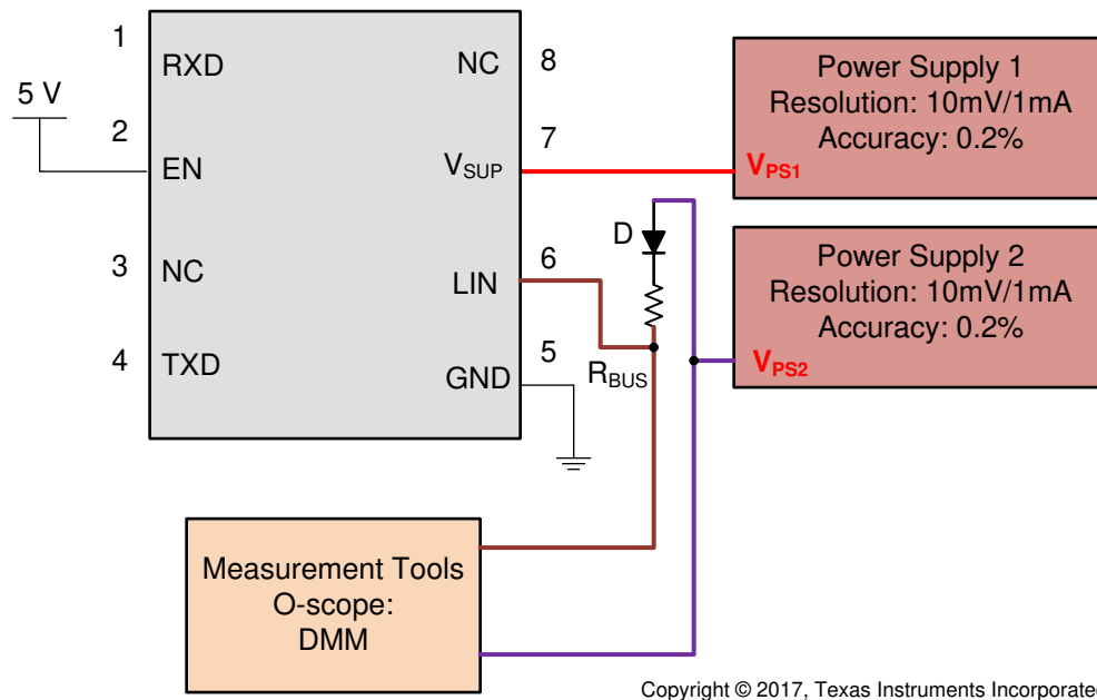
图 8-5. V<sub>SUP</sub>-NON_OP Param 11 54/56
