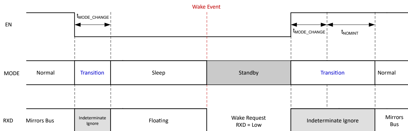
图 8-15. Mode Transitions
