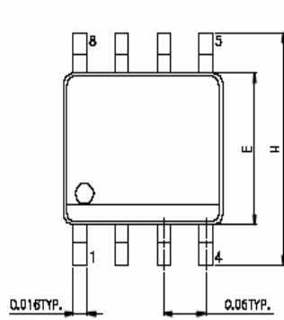
Figure 24. SOP 150 mil
