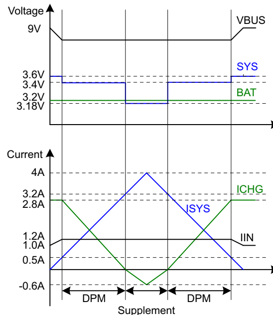
图 12. DPM Response
