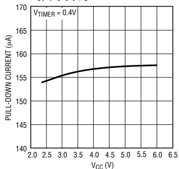
TIMER 下拉电流与电源电压的关系曲线
