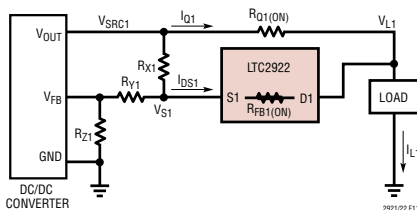
图 11：远端取样开关连接等效网络
