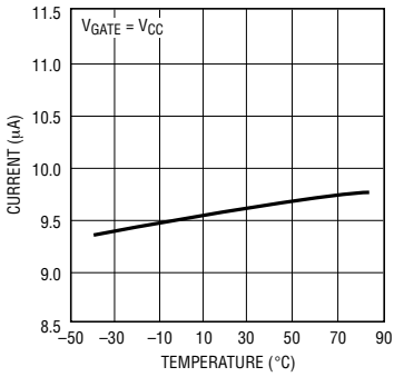
GATE 上拉电流与温度的关系曲线
