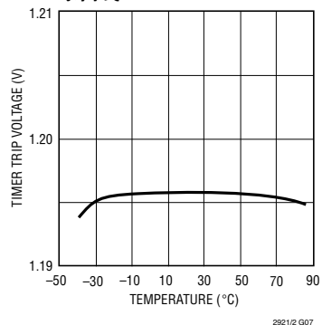
TIMER 跳变电压与温度的关系曲线
