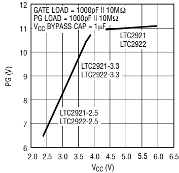
PG 电压与电源电压的关系曲线
