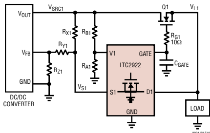
图 10：自动远端取样开关连接
