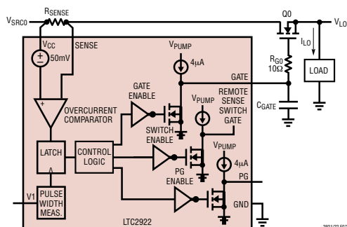
图 7：电路断路器功能电路示意图
