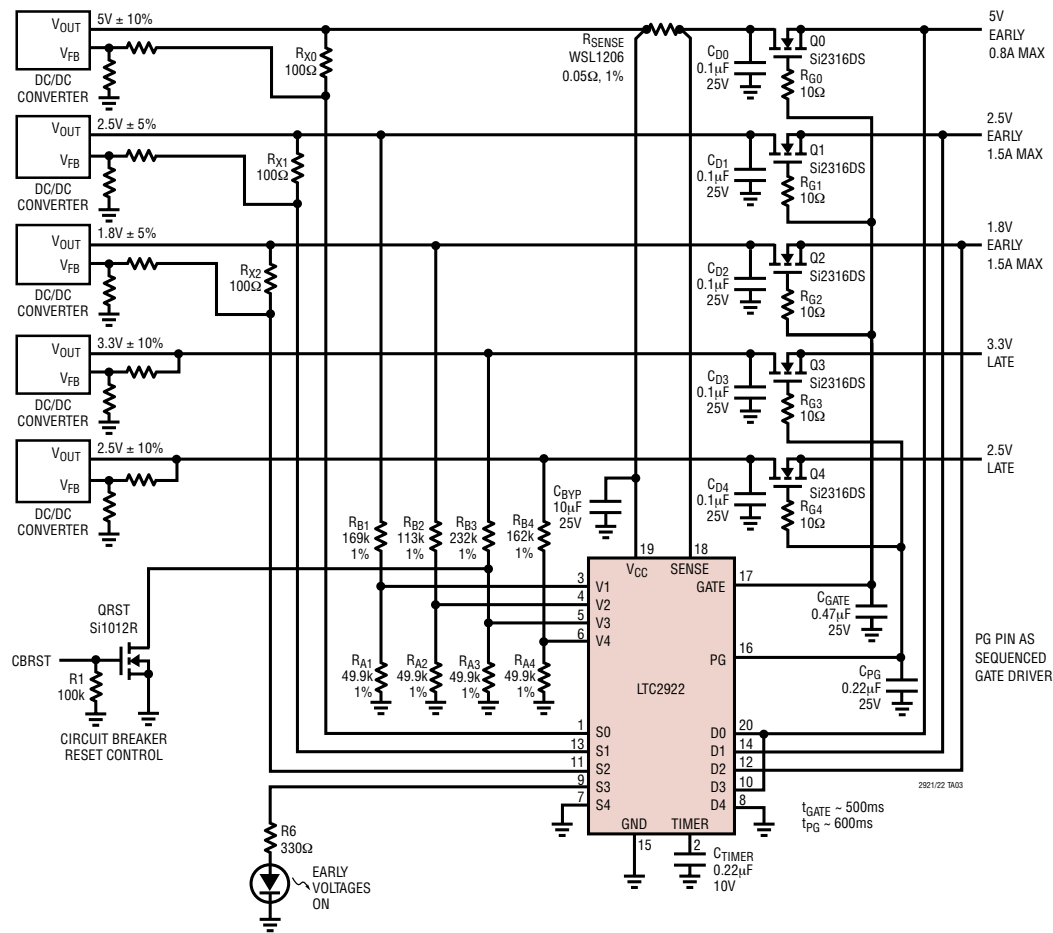
具备超前电源 LED 指示器的电源先后排序器
