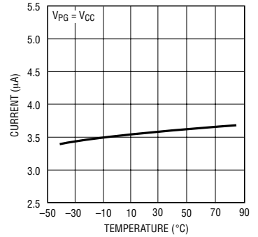
PG 上拉电流与温度的关系曲线
