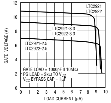
栅极电压与负载电流的关系曲线
