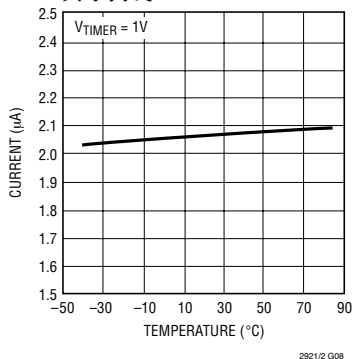
TIMER 上拉电流与温度的关系曲线
