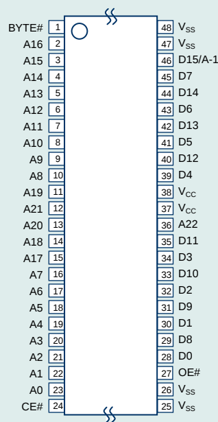
48TSOP(Type-I)
