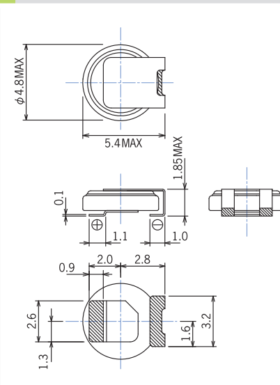
414-VE5R type
