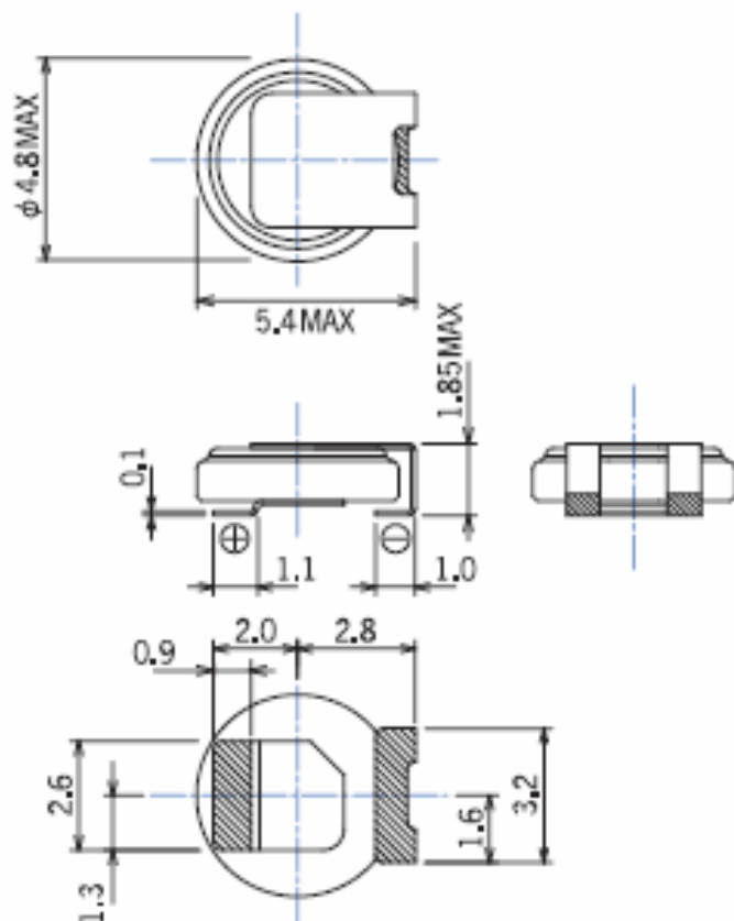
414-VE5R type
