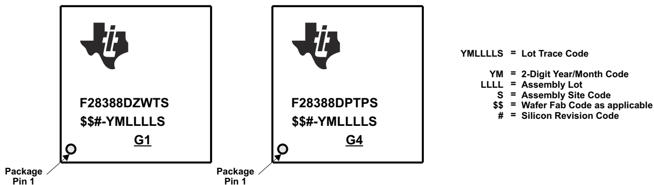
图 10-2. Package Symbolization
