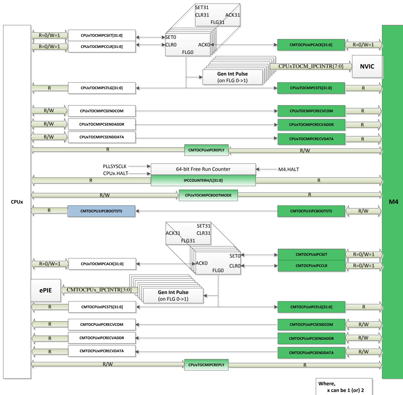
图 8-7. CPUx_to_CM IPC Module
