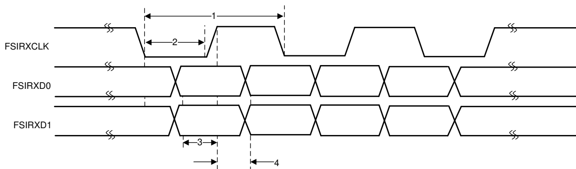
图 7-64. FSIRX Timings
