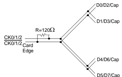
*Clock Net Wiring
