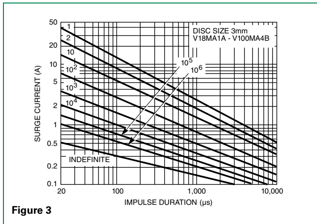
V18MA - V100MA
