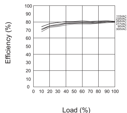
RAC04C-12DH
