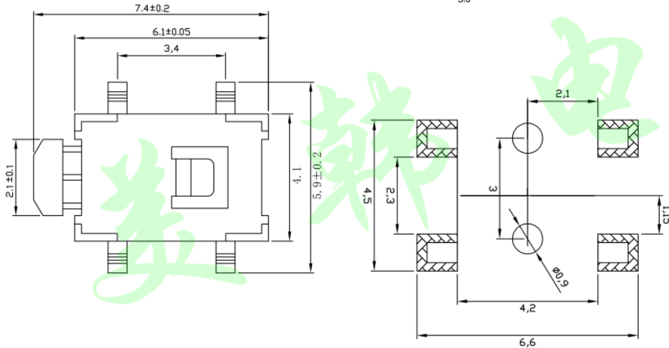
P.C.B LAND DIMENSION
