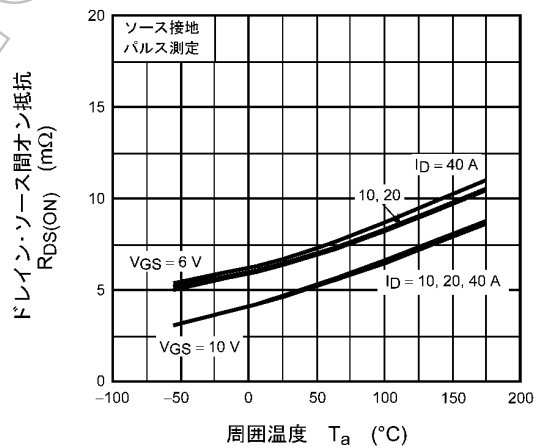
図 8.6 R_{DS(ON)} - T_a (注7)
