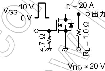
図 6.2.1 スwitching時間の測定回路例
