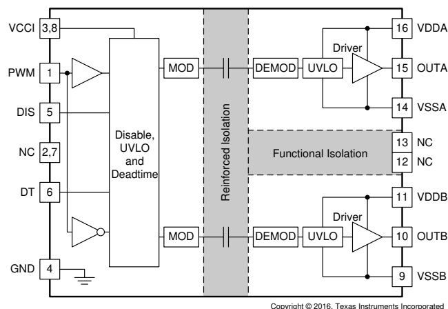
功能框图
