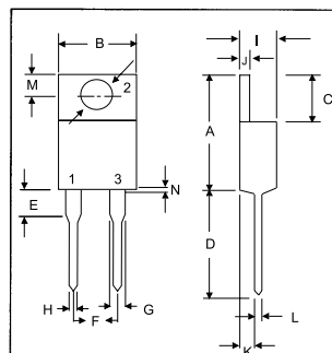
TO-220A
