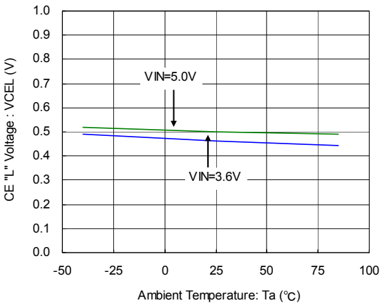
V_{OUT}=1.8V, 3.0MHz L=1.5\mu H(NR3015) , C_{IN}=4.7\mu F , C_L=10\mu F
