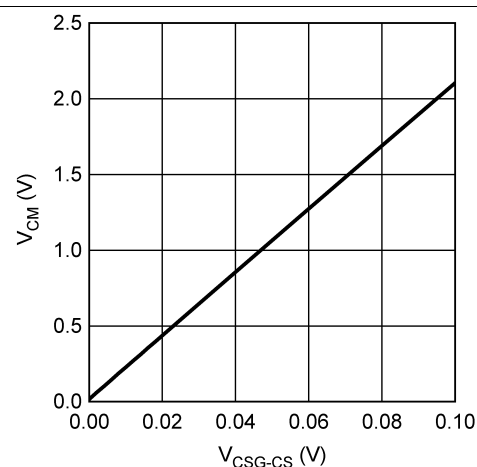
Figure 14. V_{CM} vs V_{CSG-CS}
