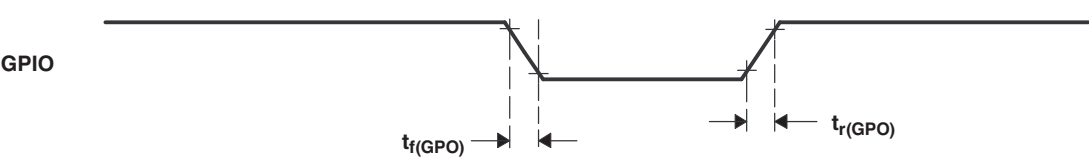
Figure 6-10. 通用输出时序
