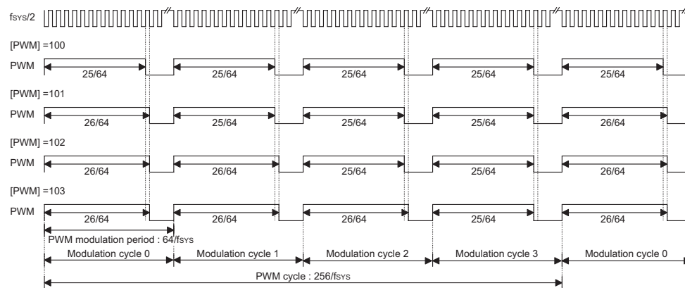
6+2 PWM Mode
