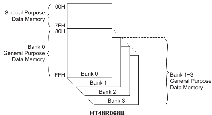
HT48R068B
