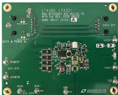
Top Side
