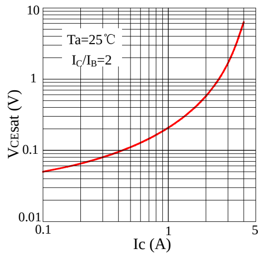
Fig3 V_{CEsat}-I_C
