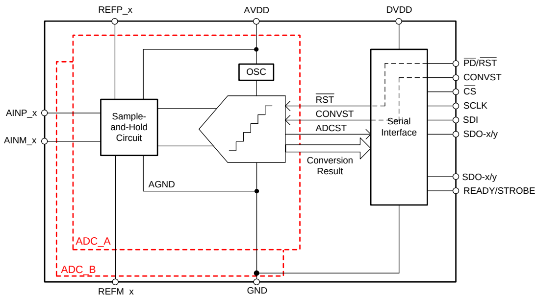
图 36. Converter Modules
