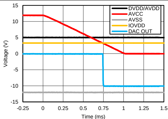
Figure 35. DAC Output With AV CC Supply Collapse
