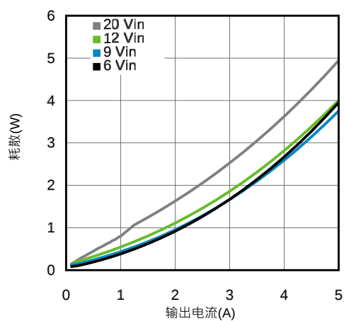
损耗1.0V输出 · 环境温度为85°C
