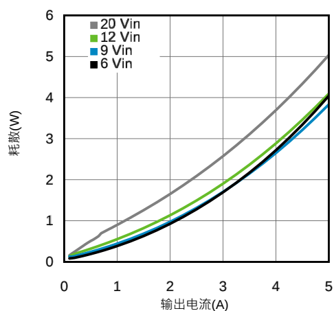
损耗1.2V输出 · 环境温度为85°C
