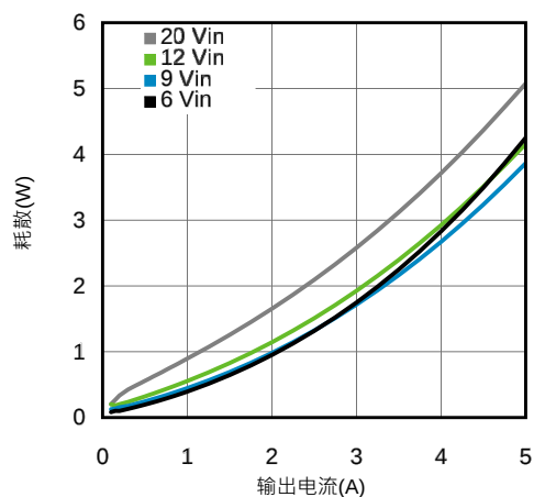
损耗1.5V输出 · 环境温度为85°C
