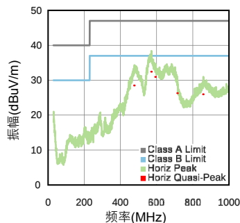
演示板(参阅AN-2125)的辐射 电磁干扰(EN55022)
