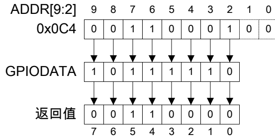
图 9-4. GPIODATA 读实例
