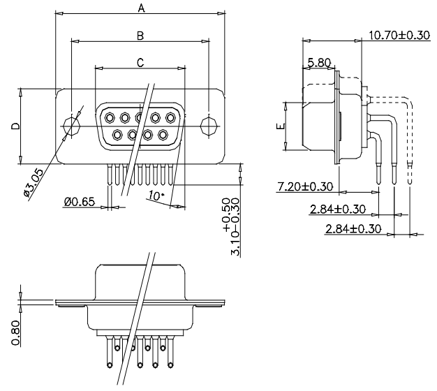
RECEPTACLE
